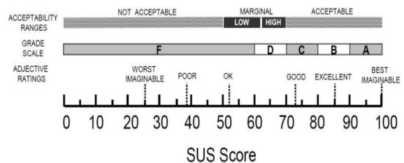
Gambar 7. SUS Skor [12]
